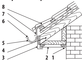
Рисунок 3.8 Карниз
