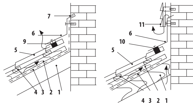
Рисунок 3.14 Поперечное примыкание кровли
