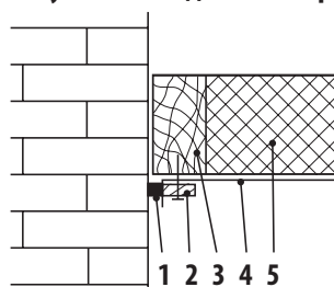
Рисунок 3.4 Соединение пароизоляционной пленки со стеной
