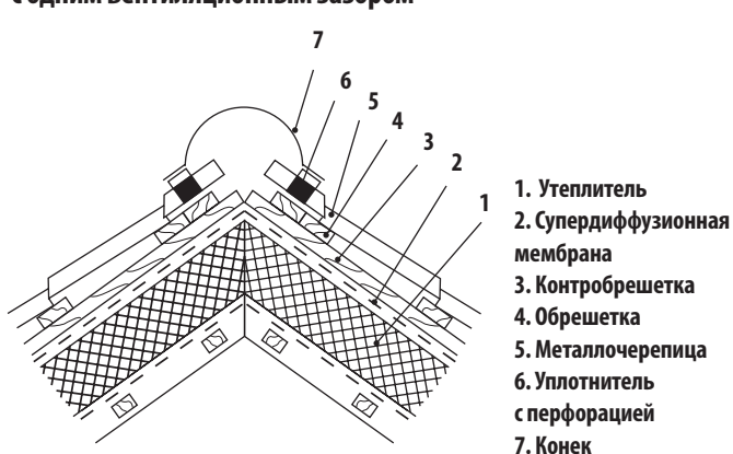
Рисунок 3.10 Конструкция конька с одним вентиляционным зазором
