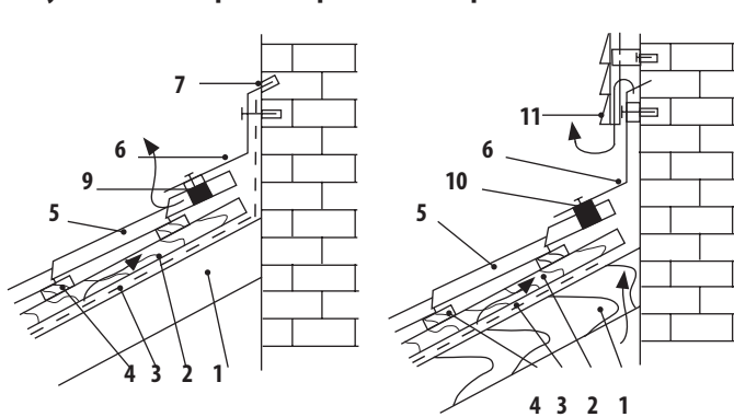
Рисунок 3.14 Поперечное примыкание кровли
